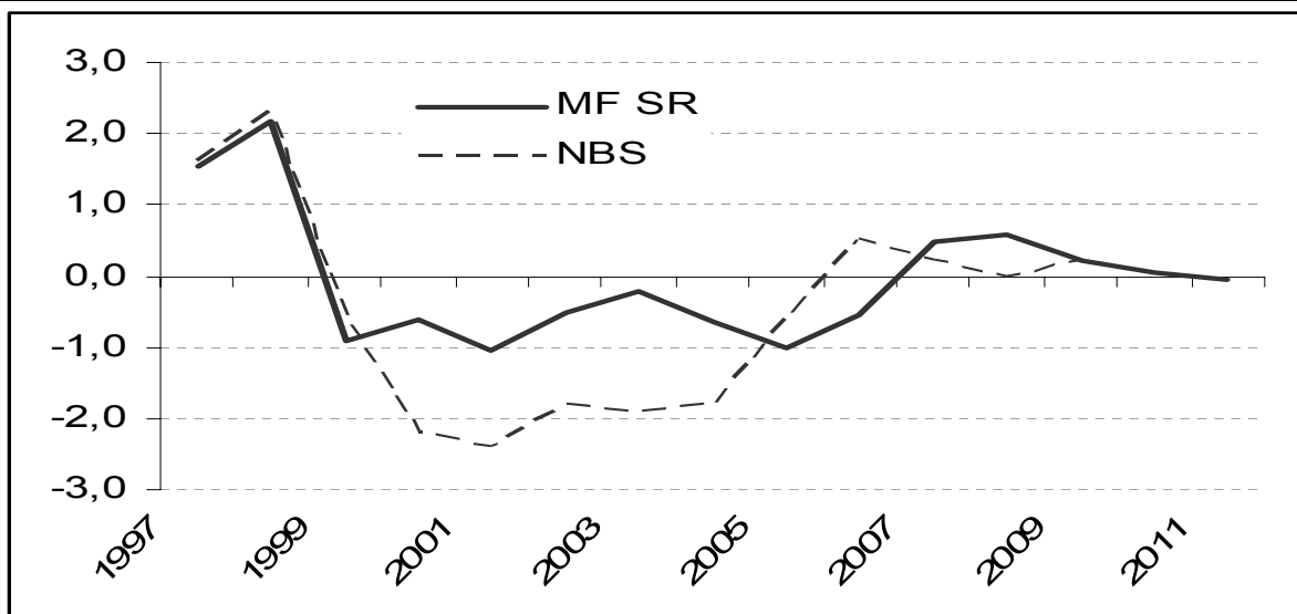
Produkčná medzera (%)
